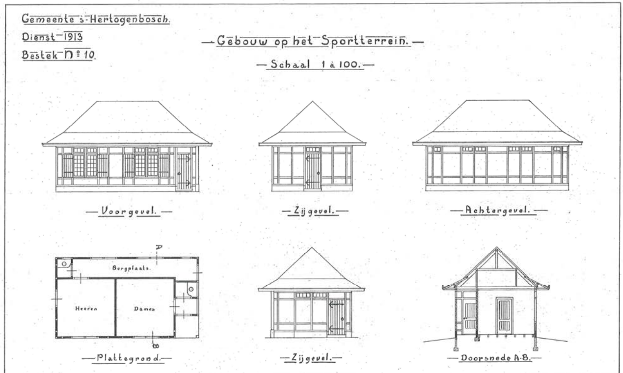
Ontwerptekening 1913, dossier Gemeentewerken nr. 779 (Erfgoed 's-Hertogenbosch).
